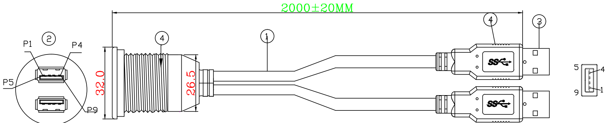
USB 3.0 A/M
