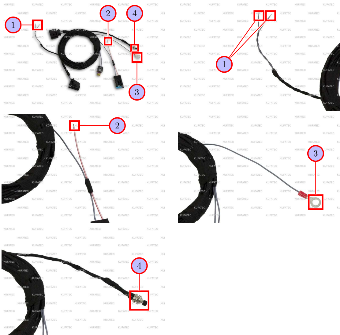
Abbildung 3: Anschluss Kabelsatz
