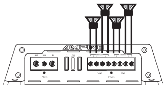
4-Kanal-Betrieb / 4-Channel configuration
