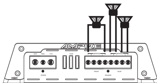
3-Kanal-Betrieb / 3-Channel configuration
