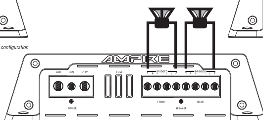
2-Kanal-Betrieb / 2-Channel configuration
