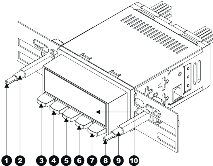
Abbildung 8 - Bedienelement
