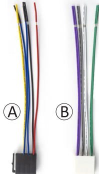
ISO-Anschlusskabel A) Strom- B) Lautsprecherkabelbaum
