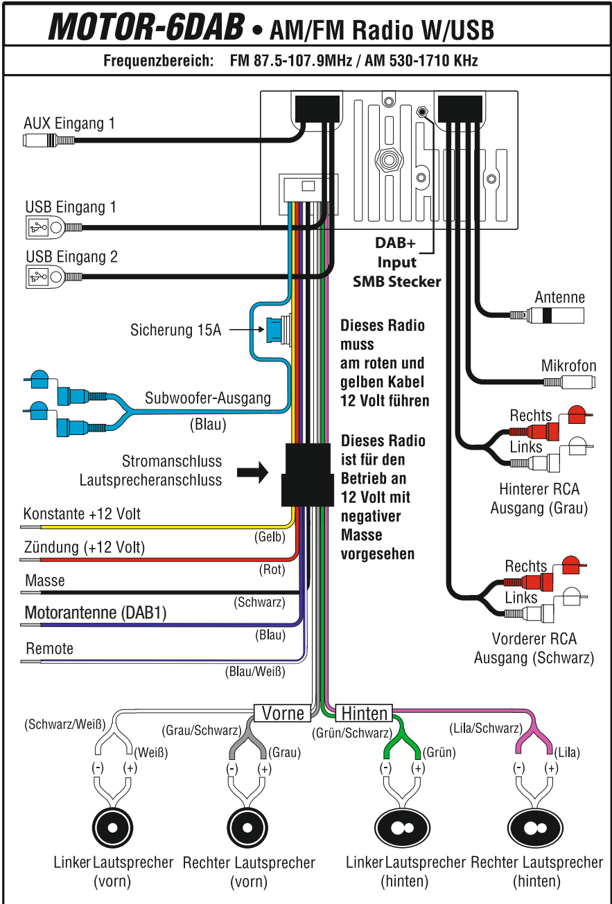
Abbildung 7 - Kabelplan
